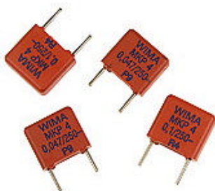
Abb.: WIMA-Kondensator MKP4 in 250V Spannungsfestigkeit
